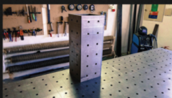
3D upínací věž - UNI.7121
